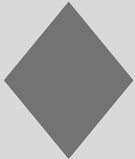
Rhombus
